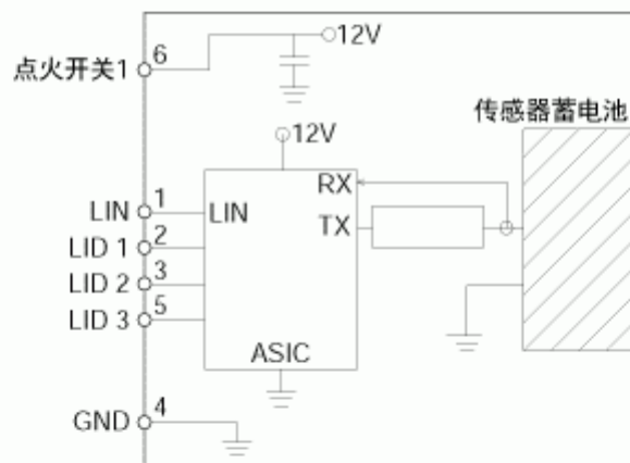
电路图
